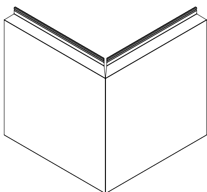
Elemento d'angolo piegato a 90° [solo su XLINE] 90° folded corner element [on XLINE only]
